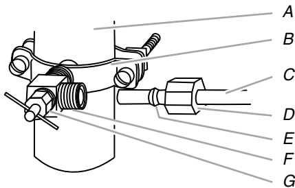
A. Canalisation d'eau froide B. Bride de tuyau C. Tube en cuivre D. Écrou de serrage E. Bague de compression F. Robinet d'arrêt G. Écrou de compression
